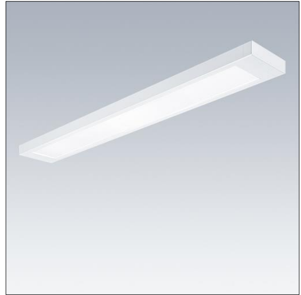
TLG_PNCH_F_LRO_surface_on_PDB.jpg
